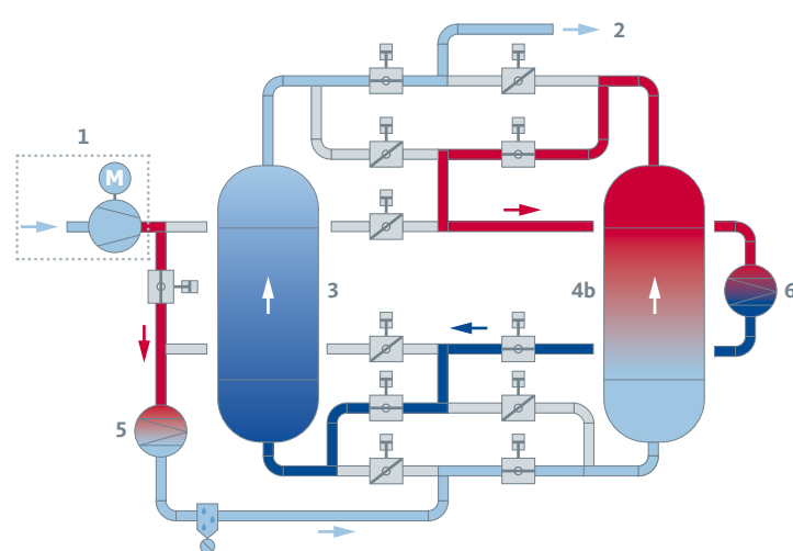
Fase di raffreddamento
