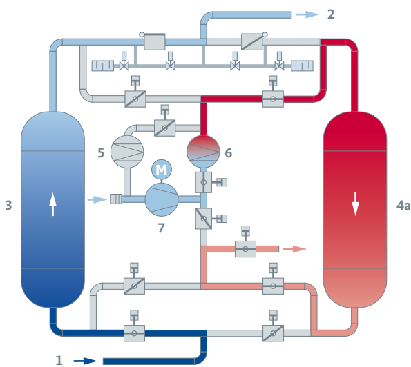
Fase di deadsorbimento
