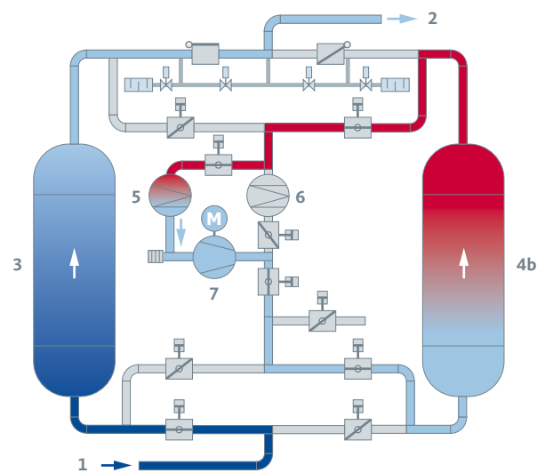
Fase di raffreddamento
