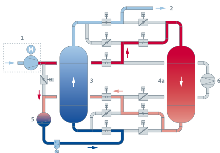
Fase di deadsorbimento
